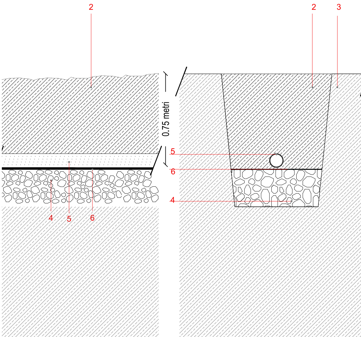
PARTICOLARE SEZIONE CONDOTTA DI SUB-IRRIGAZIONE RAPP. 1:50
