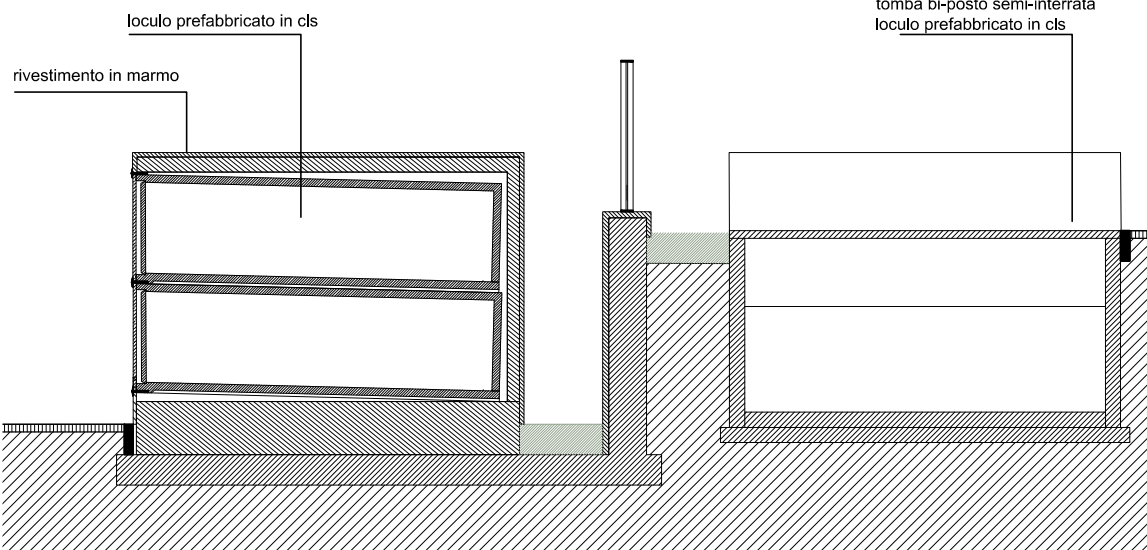
Sezione CC
