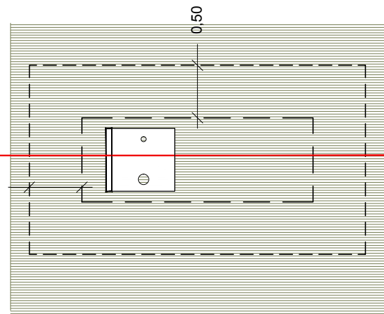
Pianta 1:50
