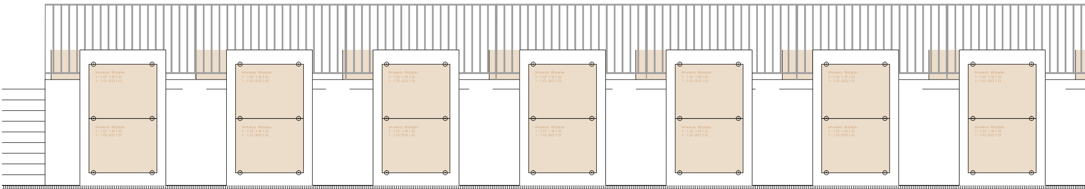
Prospetto A-A
