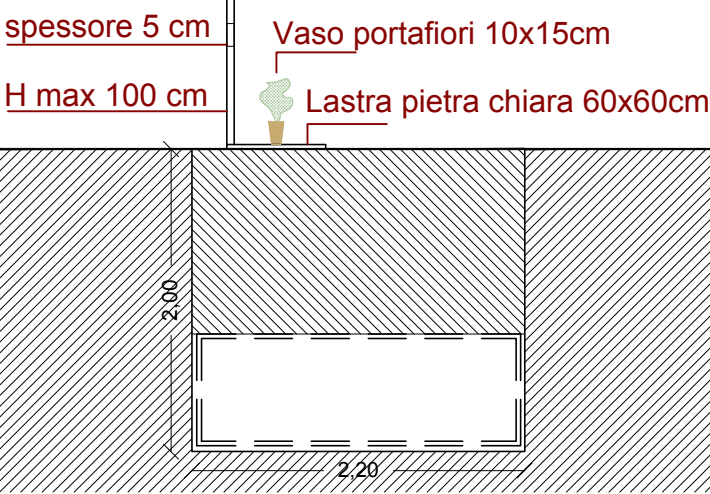
Sezione longitudinale 1:50
