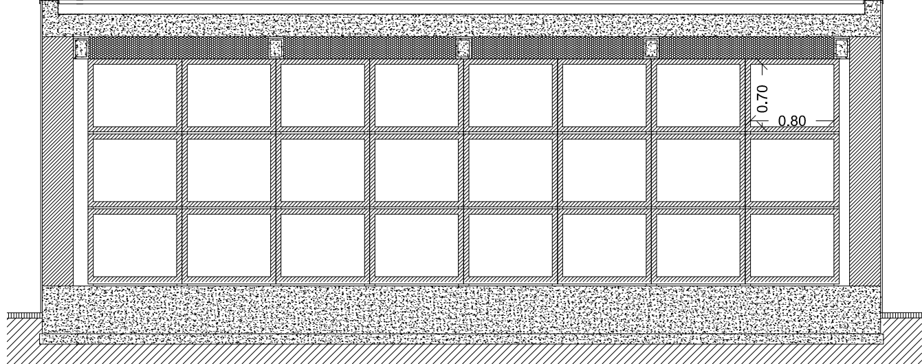
Sezione A-A
