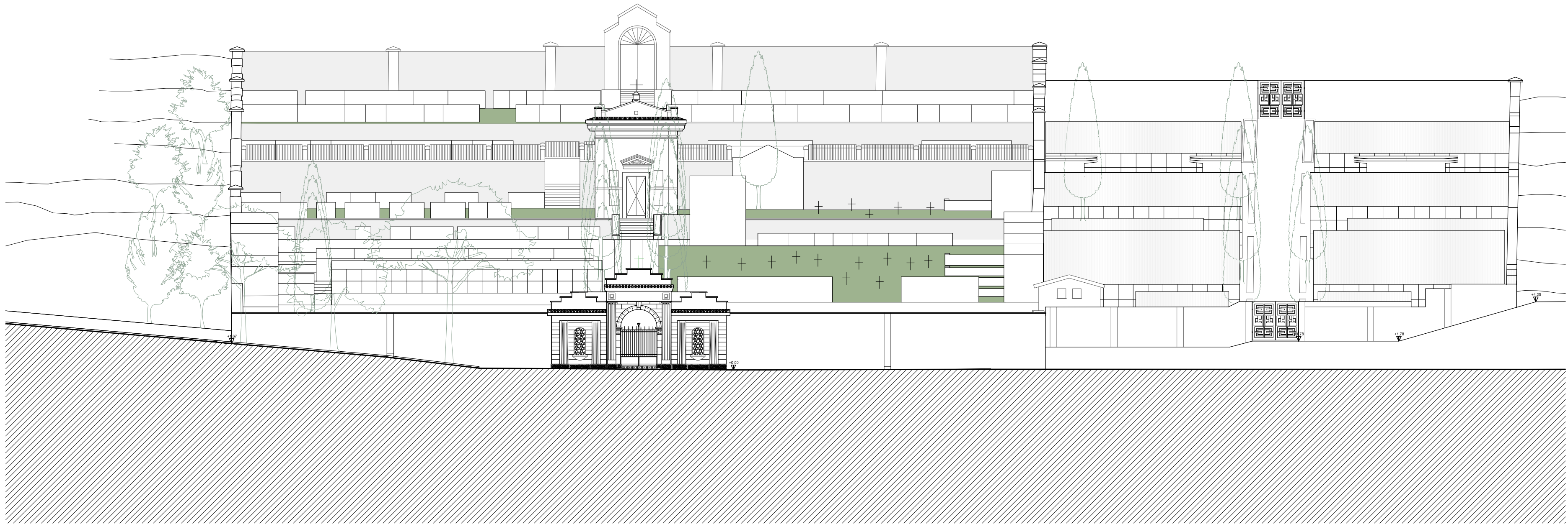
PROFILO A-A
